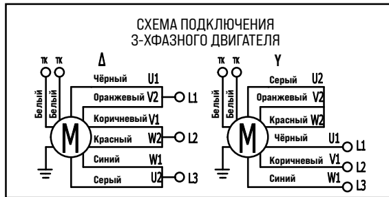
СХЕМА ПОДКЛЮЧЕНИЯ:
