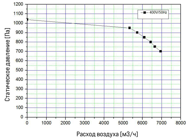
КРИВАЯ РАСХОДА:
