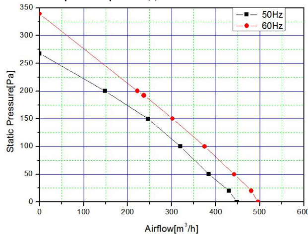
Кривая расхода:
