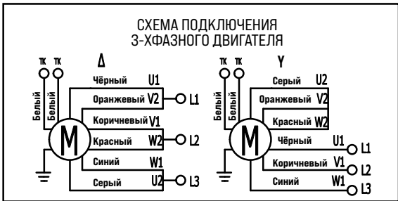
СХЕМА ПОДКЛЮЧЕНИЯ:
