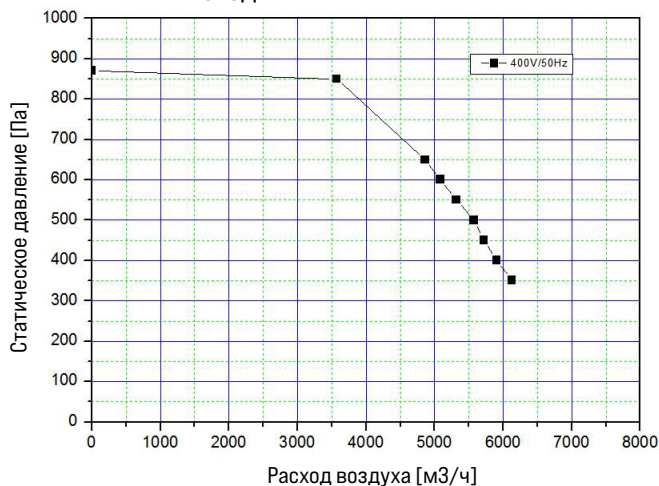
КРИВАЯ РАСХОДА:
