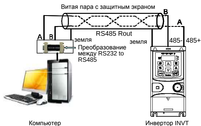
Рис. 7.1 Подключение по протоколу RS485
