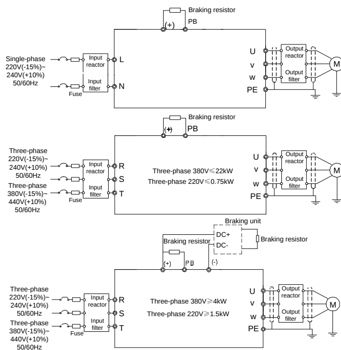
Рис. 3.3 Монтажная схема силовой цепи
