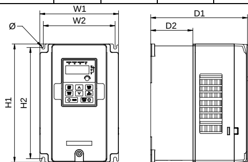
Рис. В.3 Настенное крепление инверторов 3 ф. 380 В мощностью 4~37 кВт и 3 ф. 220 В мощностью 1.5~7.5 кВт
