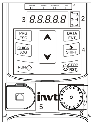
Рис. 4.1 Пленочная клавиатура
