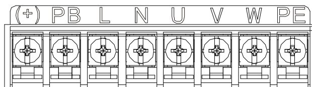
Рис. 3.4 Клеммы силовой цепи однофазного инвертора
