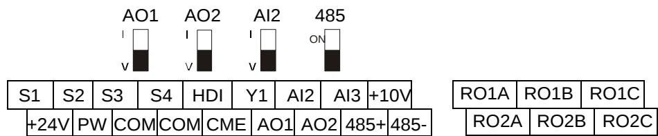
Рис. 3.10 Клеммы цепей управления
