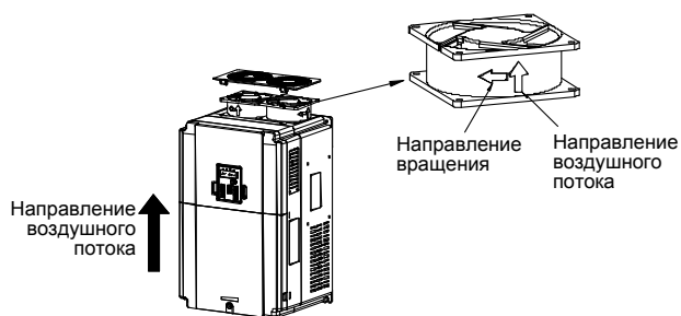
Рис. 6.1 Монтаж вентилятора в инверторах: 3 фазы / 380 В, мощностью более 4 кВт
