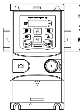
крепление на монтажную рейку
