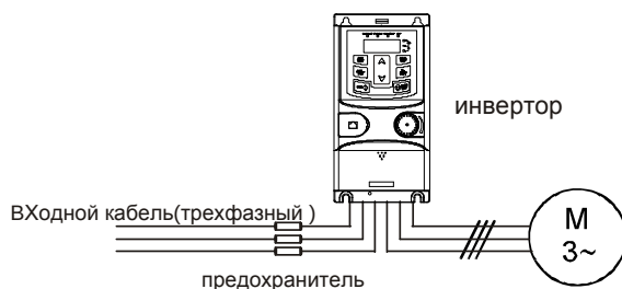
Рис. 3.14 Расположение предохранителей
