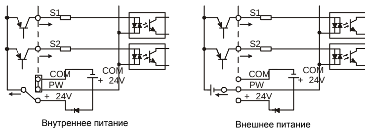
Рис. 3.13 Режимы PNP
