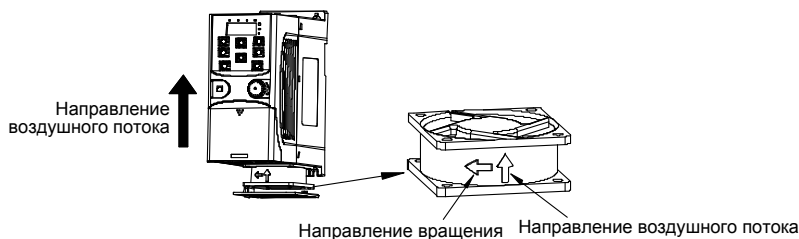
Монтаж вентилятора в инверторах: 1 фаза / 220 В, мощностью менее 2,2 кВт
