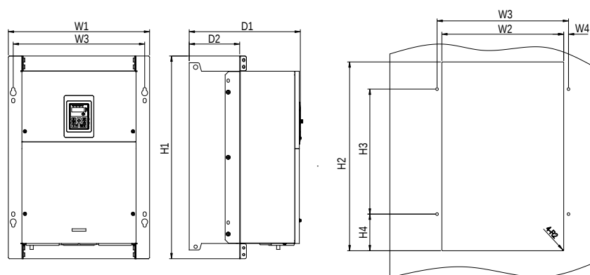
Рис. В.7 Фланцевое крепление инверторов 3 ф. 380 В мощностью 90~110 кВт
