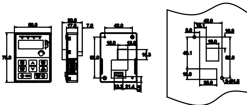
Габаритно-присоединительный чертеж
