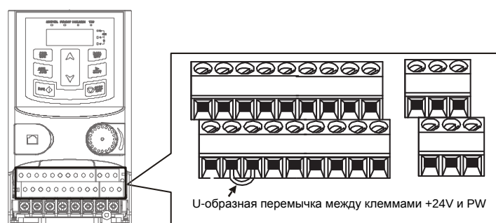
Рис. 3.11 U-образная перемычка
