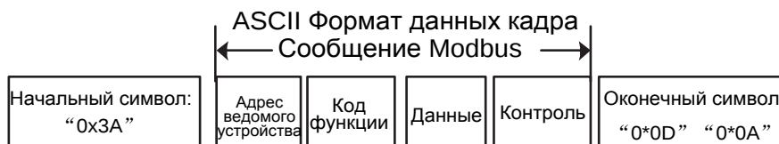
Стандартная структура кадра ASCII
