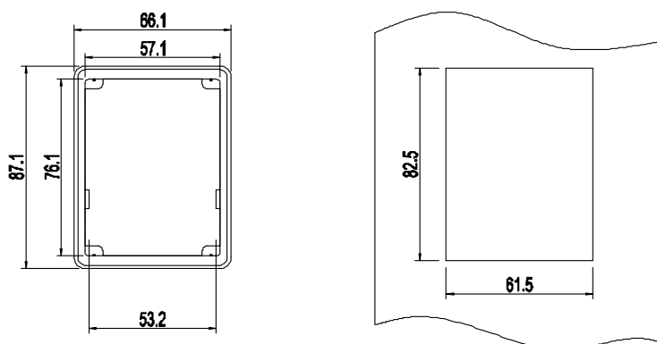
Монтажный кронштейн
