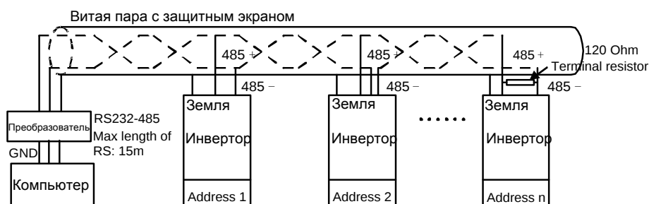
Рис. 7.2 Схема последовательного подключения
