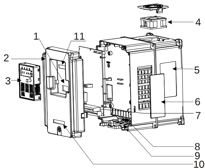
Рис. 2.4 Конструктивное исполнение изделия (3 фазы, 380 В, \geq 4 кВт)
