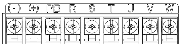
Рис. 3.7 Клеммы силовой цепи трехфазного инвертора (мощностью 30–37 кВт)
