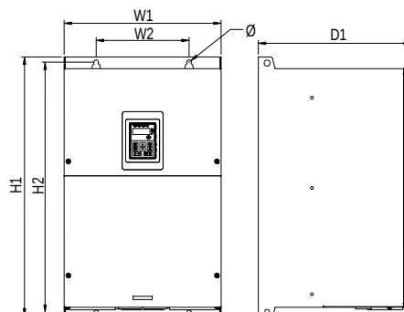
Рис. В.5 Настенное крепление инверторов 3 ф. 380 В мощностью 90~110 кВт
