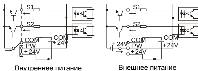
Рис. 3.12 Режимы NPN
