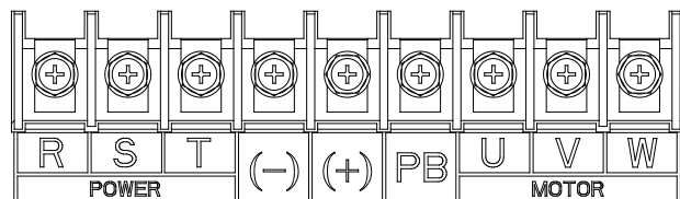
Рис. 3.8 Клеммы силовой цепи трехфазного инвертора (мощностью 45–110 кВт)
