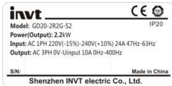
Рис. 2.1 Заводская табличка
