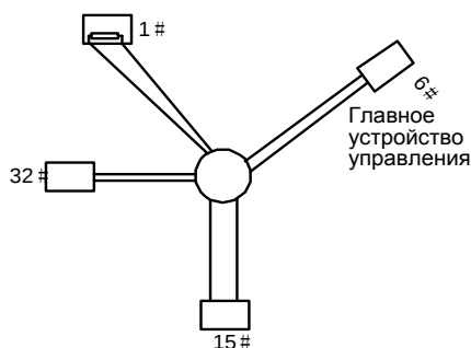
Рис. 7.3 Подключение по схеме «Звезда»
