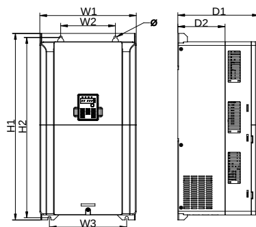
Рис. В.4 Настенное крепление инверторов 3 ф. 380 В мощностью 45~75 кВт
