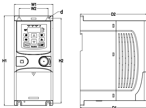
Рис. В.1 Настенное крепление инверторов мощностью 0.75~2.2 кВт
