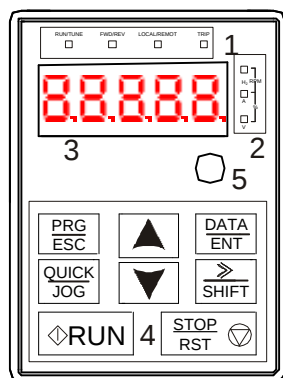
Рис. 4.2 Внешняя клавиатура
