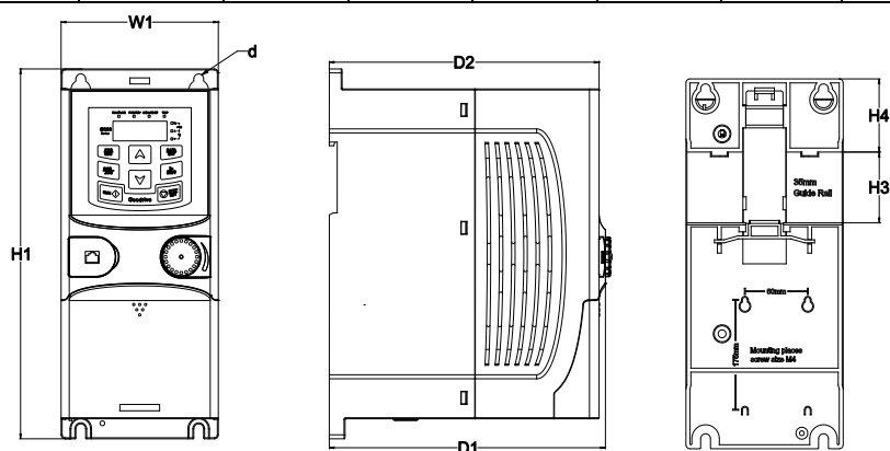
Рис. В.2 Установка на монтажную рейку инверторов 1 ф. 220 В / 3 ф. 380 В ( \leq 2.2 кВт) и 3 ф. 220 В ( \leq 0.75 кВт)
