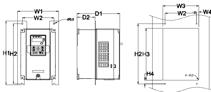
Рис. В.6 Фланцевое крепление инверторов 3 ф. 380 В мощностью 4~75 кВт и 3 ф. 220 В мощностью 1.5~7.5 кВт
