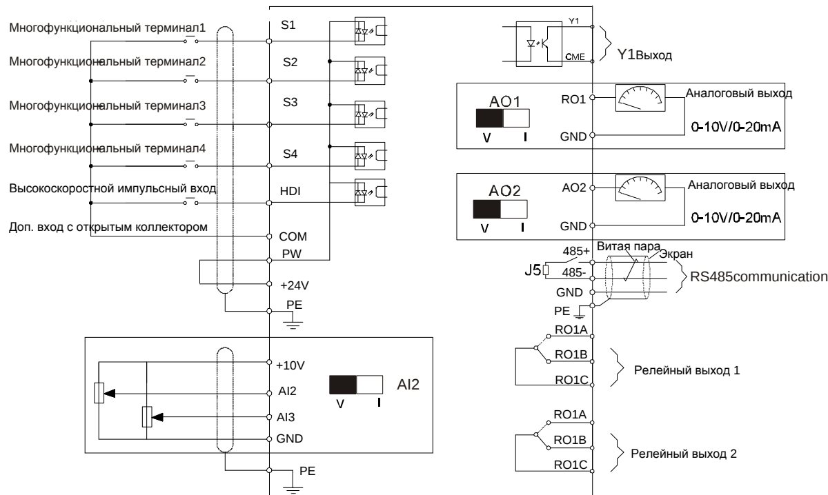
Рис. 3.9 Проводка цепей управления
