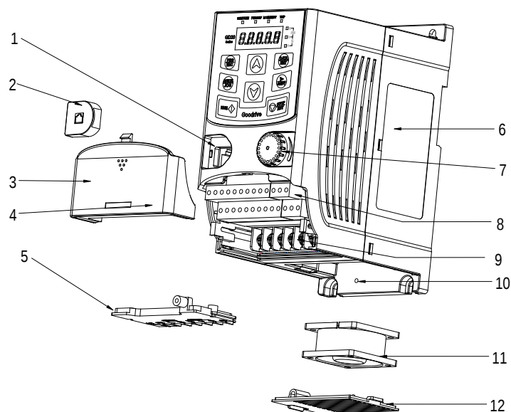
Рис. 2.3: Конструктивное исполнение изделия (3 фазы, 380 В, \leq 2,2 кВт)
