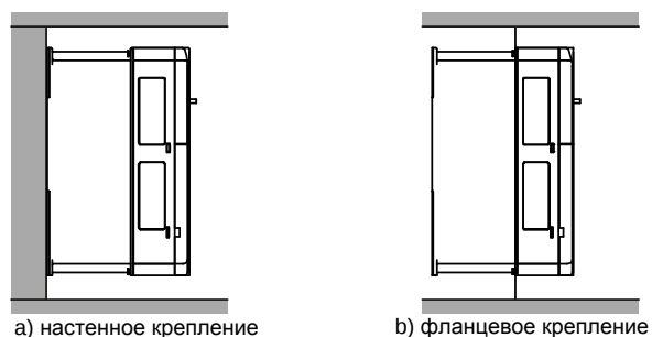
Рис. 3.2 Установка инвертора
