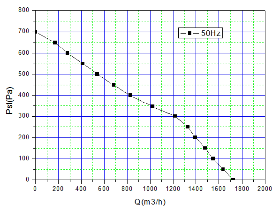
Кривая расхода:
